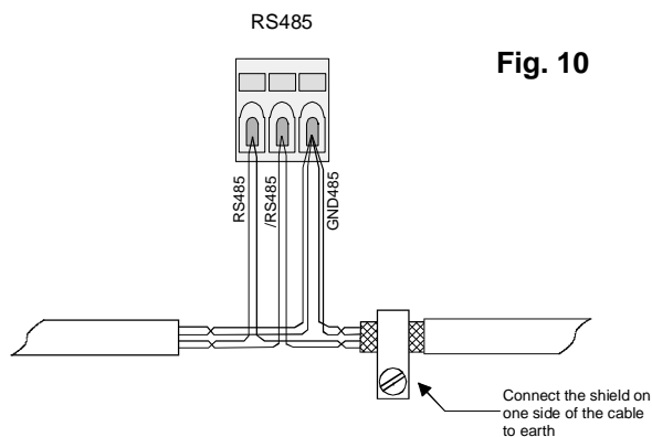
RS-485
